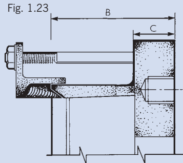
Tapped flange
