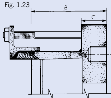
Tapped flange
